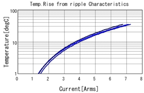
GRM21BC80E107ME15 Temp. rise ■ 50kHz ■ 200kHz ■ 400kHz
