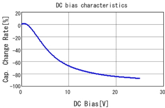
■ GRM21BC71E106ME11 C-DC bias capchange, 25.0degC, AC1V
