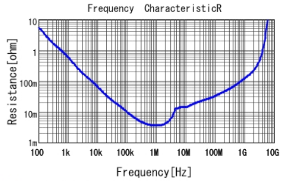
■ GRM21BB31E106KA73 R DCOV, 20degC
