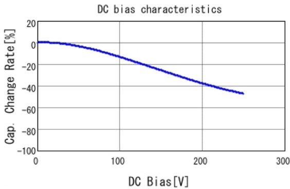
■ GRM188R72E221KW07 C-DC bias capchange, 25.0degC, AC1V
