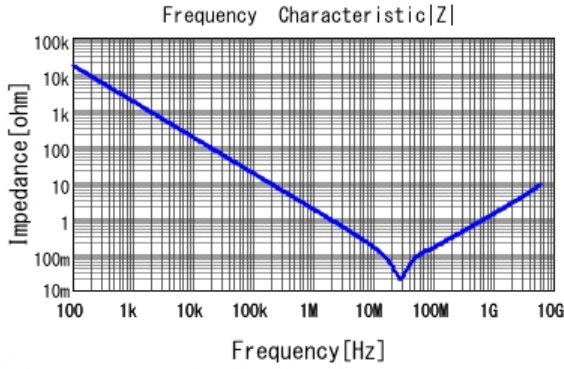
■ GRM155R71H104ME14 |Z| DCOV, 25degC
