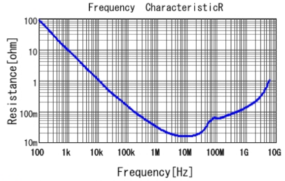
■ GRM155R71H104ME14 R DCOV, 25degC
