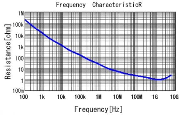
■ GRM033B11E101KA01 R DCOV, 20degC
