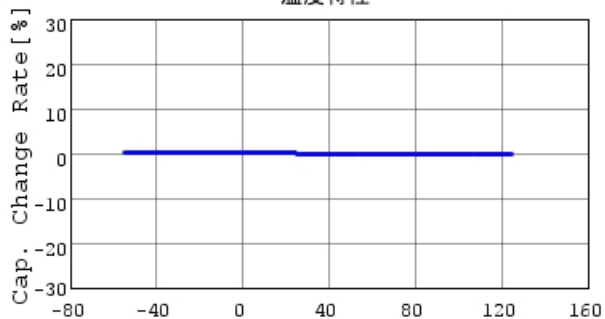
温度特性
