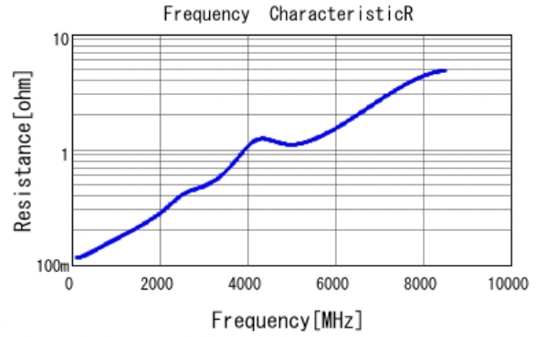
■ GRM0332C1H820JA01 R DCOV, 20degC
