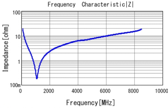
■ GRM0332C1H820JA01 |Z| DCOV, 20degC
