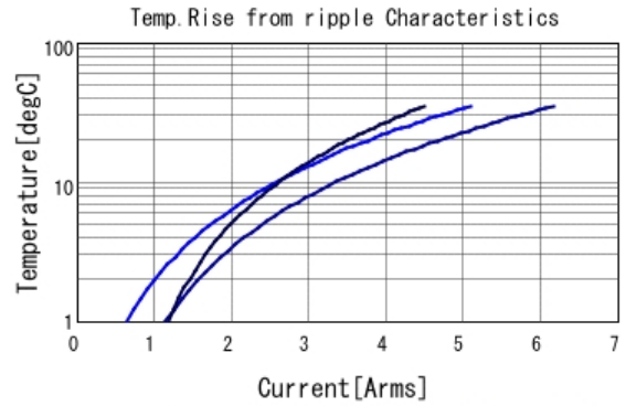
GRJ32ER71C226KE11 Temp. rise ■ 80kHz ■ 400kHz ■ 800kHz
