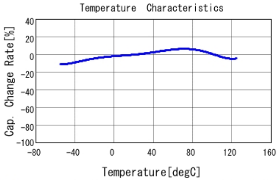
■ GRJ32ER71C226KE11 C-Temp. capchange, DCO. 0V, ACO. 5Vrm
