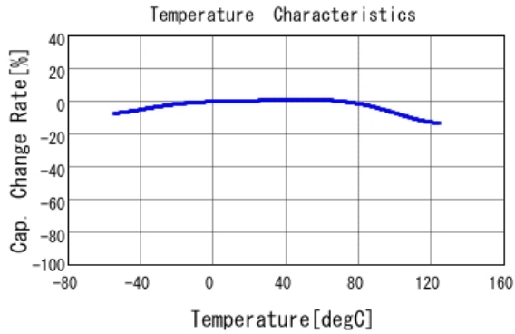
■ GRJ32ER71A476KE11 C-Temp. capchange, DCO. 0V, ACO. 5Vrm
