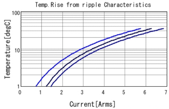
GRJ32ER71A476KE11 Temp. rise ■ 60kHz ■ 300kHz ■ 600kHz
