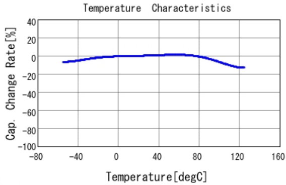
■ GRJ32ER70J476KE11 C-Temp. capchange, DCO. 0V, ACO. 5Vrm
