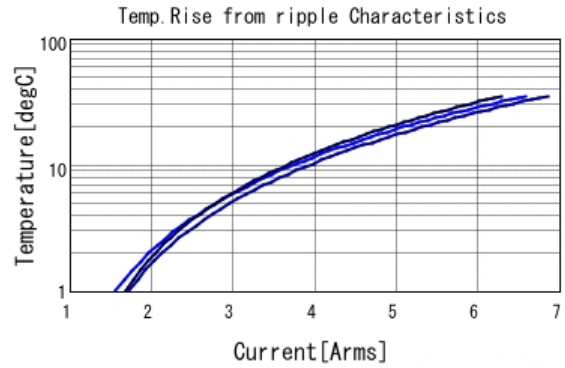
GRJ32ER70J476KE11 Temp. rise ■ 60kHz ■ 300kHz ■ 600kHz
