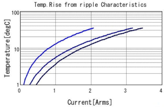
GRJ188R70J225KE11 Temp. rise ■ 100kHz ■ 500kHz ■ 1MHz
