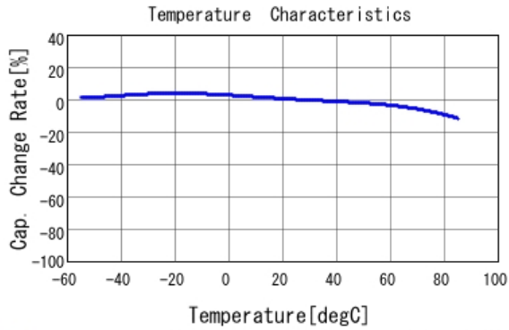
■ GRJ188R60J106ME11 C-Temp. capchange, DCO. 0V, ACO. 5Vrm
