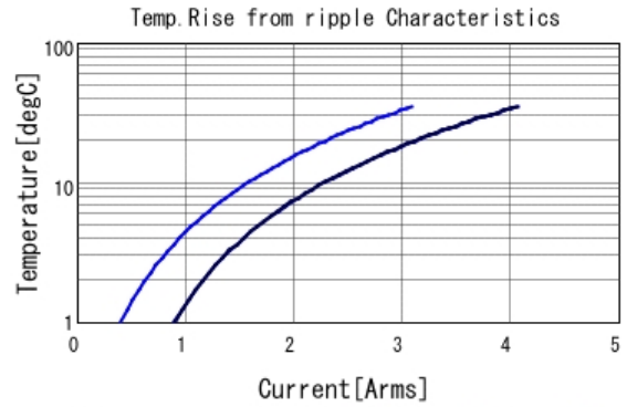
GRJ188R60J106ME11 Temp. rise ■ 80kHz ■ 400kHz ■ 800kHz
