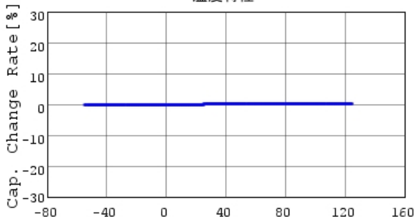
温度特性
