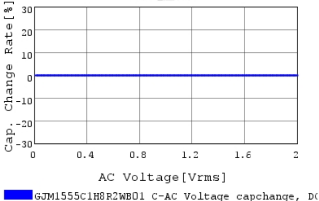
交流电压特性
