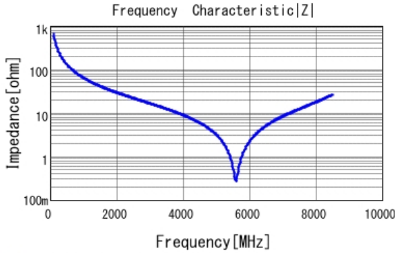
■ GCQ1555C1H2R4WB01 |Z| DC0V, 25degC
