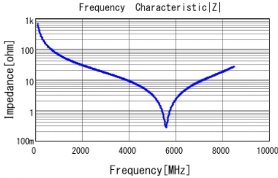
■ GCQ1555C1H2R4BB01 |Z| DC0V, 25degC
