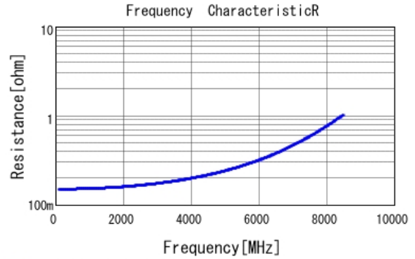
■ GCQ1555C1H2R4BB01 R DC0V, 25degC
