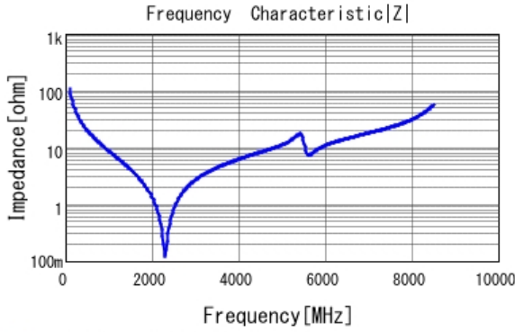
■ GCQ1555C1H150JB01 |Z| DC0V, 25degC
