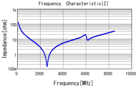
■ GCQ1555C1H120JB01 |Z| DC0V, 25degC
