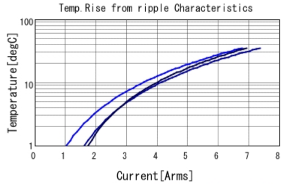
■ GCM32EC71A476KE02 Temp. rise ■ 60kHz ■ 300kHz ■ 600kHz
