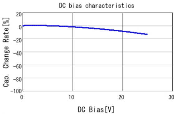
GCM21BR71E224KA37 C-DC bias capchange, 25.0degC, AC1.
