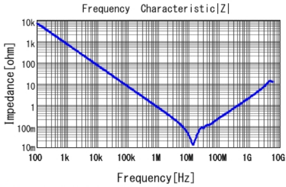
GCM21BR71E224KA37 |Z| DC0V, 25degC
