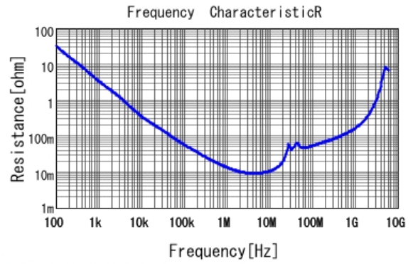
GCM21BR71E224KA37 R DC0V, 25degC
