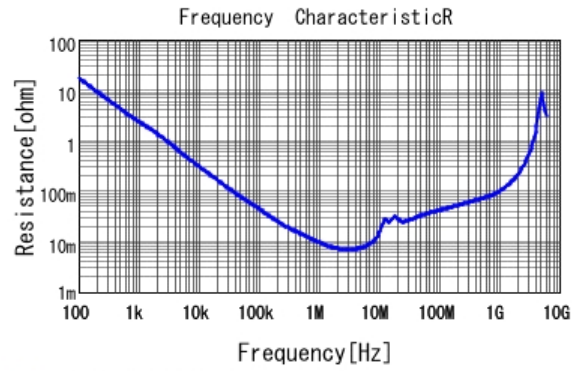
■ GCM21BR71E155KA54 R DC0V, 25degC
