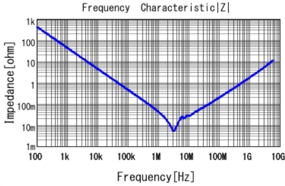
■ GCM21BC71E475KE36 |Z| DC0V, 25degC
