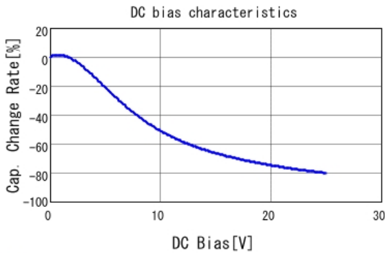
■ GCM21BC71E475KE36 C-DC bias capchange, 25.0degC, AC1V
