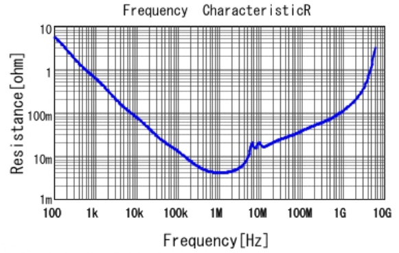
■ GCM21BC71E475KE36 R DC0V, 25degC
