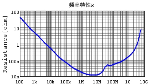
GCM188R71E224KA55 R DCOV, 25degC
