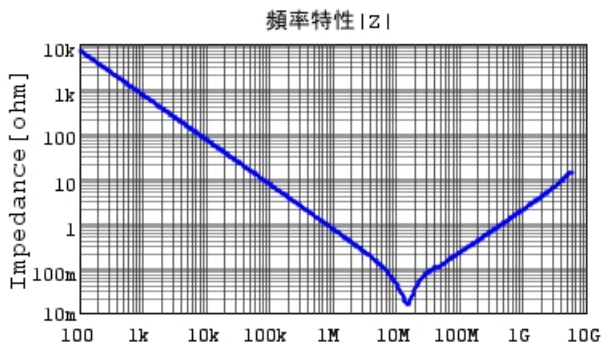
GCM188R71E224KA55 |Z| DCOV, 25degC
