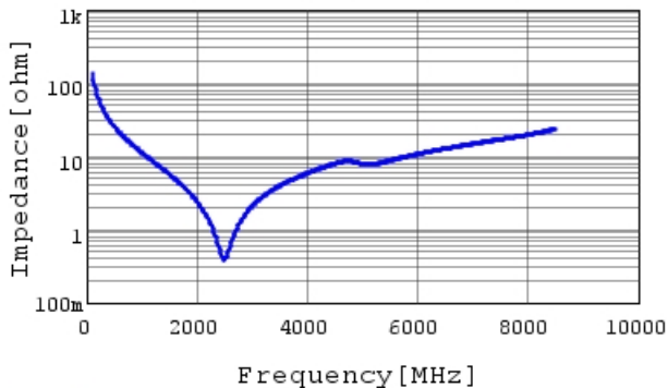
频率特性 |Z|
