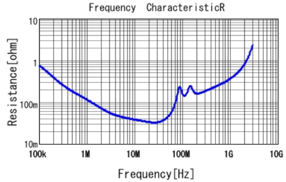
■ GCJ32DR73A223KXJ1 R DC0V, 25degC
