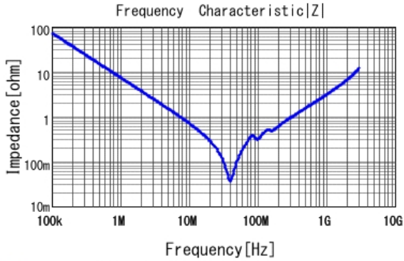
■ GCJ32DR73A223KXJ1 |Z| DC0V, 25degC
