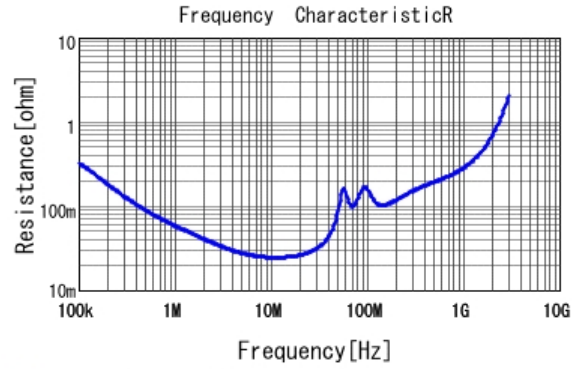
■ GCJ32DR72J473KXJ1 R DC0V, 25degC
