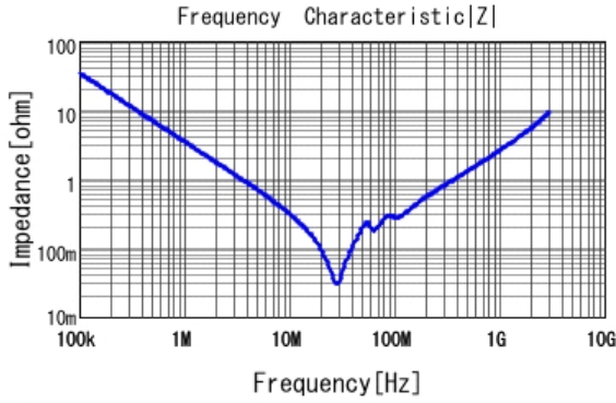
■ GCJ32DR72J473KXJ1 |Z| DC0V, 25degC
