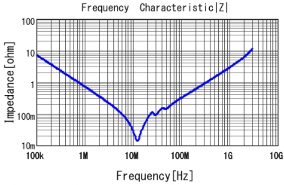
■ GCJ32DR72E224KXJ1 |Z| DC0V, 25degC
