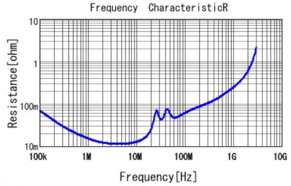
■ GCJ32DR72E224KXJ1 R DC0V, 25degC
