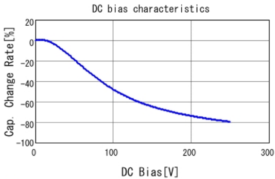
■ GCJ32DR72E224KXJ1 C-DC bias capchange, 25.0degC, AC1V
