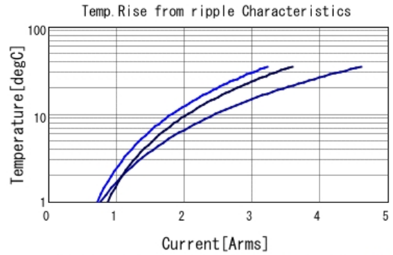
GCJ32DL8EL225KA07 Temp. rise ■ 100kHz ■ 500kHz ■ 1MHz
