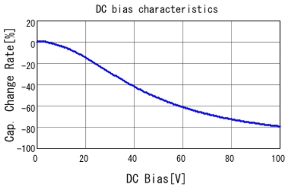
■ GCJ32DL8EL225KA07 C-DC bias capchange, 25.0degC, AC1.
