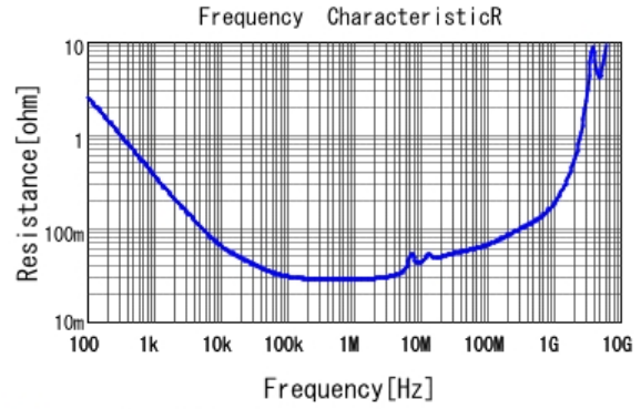
■ GCJ32DL8EL225KA07 R DC0V, 25degC
