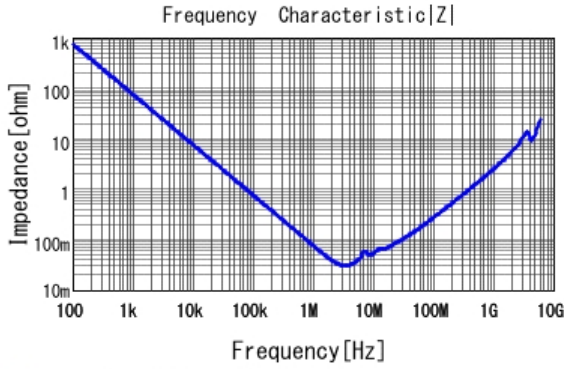
■ GCJ32DL8EL225KA07 |Z| DC0V, 25degC
