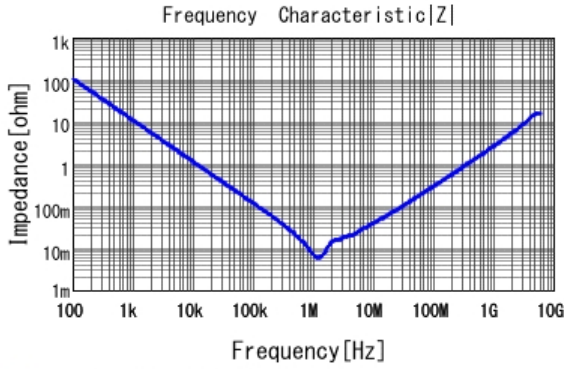
■ GCJ31CR71A226KE01 |Z| DC0V, 25degC
