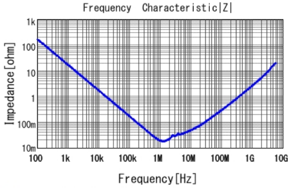
■ GCJ31CC71E106MA15 |Z| DCOV, 25degC
