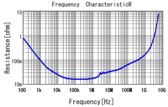
■ GCJ31CC71E106MA15 R DCOV, 25degC
