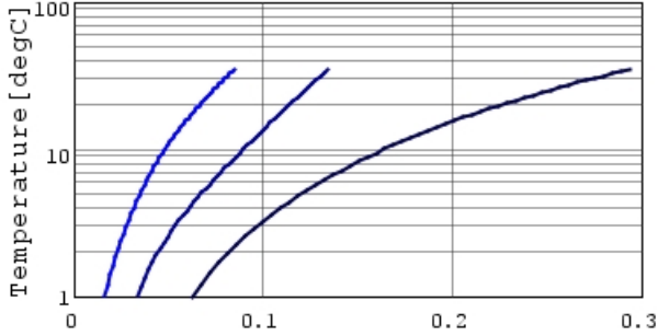
GCJ31BR73A472KXJ1 Temp.rise — 30kHz —
