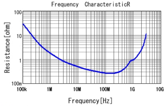
■ GCJ31BR73A152KXJ1 R DC0V, 25degC
