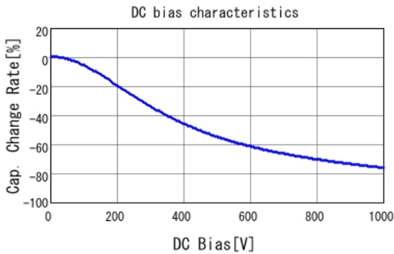
■ GCJ31BR73A152KXJ1 C-DC bias capchange, 25.0degC, AC1V
