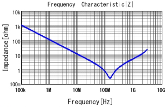
■ GCJ31BR73A152KXJ1 |Z| DC0V, 25degC
