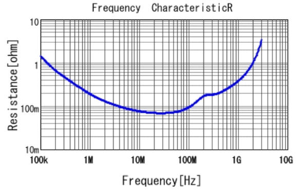
■ GCJ21BR72E153KXJ3 R DC0V, 25degC
