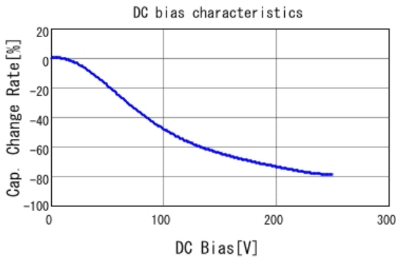
■ GCJ21BR72E153KXJ3 C-DC bias capchange, 25.0degC, AC1V
