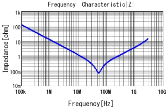
■ GCJ21BR72E153KXJ3 |Z| DC0V, 25degC
