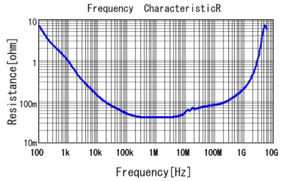
■ GCJ21BR71C105KA01 R DCOV, 25degC
