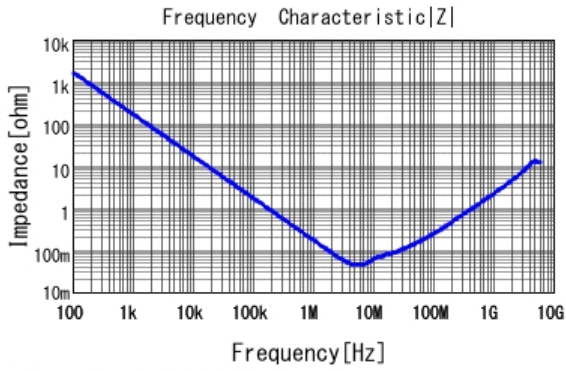
■ GCJ21BR71C105KA01 |Z| DCOV, 25degC
