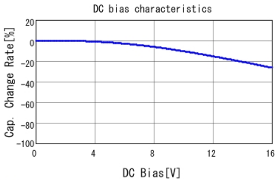
■ GCJ21BR71C105KA01 C-DC bias capchange, 25.0degC, AC1.
