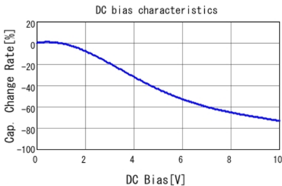
■ GCJ21BR71A106KE01 C-DC bias capchange, 25.0degC, AC1V
