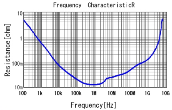
■ GCJ21BR71A106KE01 R DC0V, 25degC
