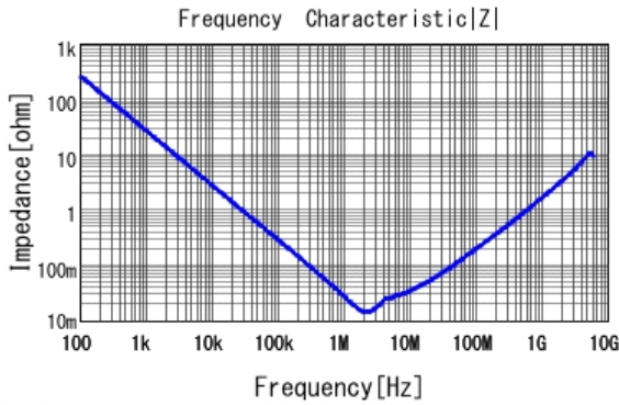
■ GCJ21BR71A106KE01 |Z| DC0V, 25degC
