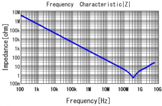
■ GCJ219R72A471KA01 |Z| DCOV, 25degC
