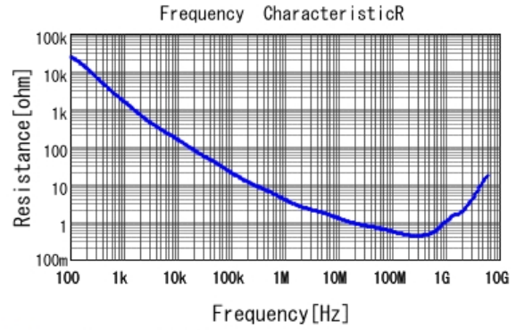
■ GCJ219R72A471KA01 R DCOV, 25degC
