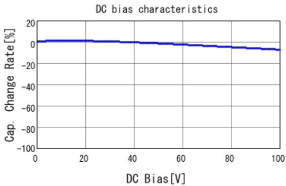
■ GCJ219R72A471KA01 C-DC bias capchange, 25.0degC, AC1.
