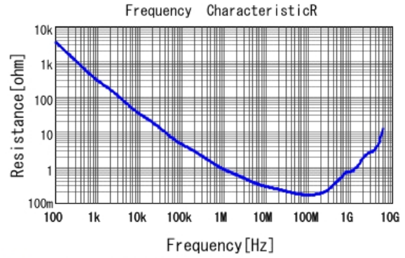
■ GCJ216R71H222KA01 R DCOV, 25degC
