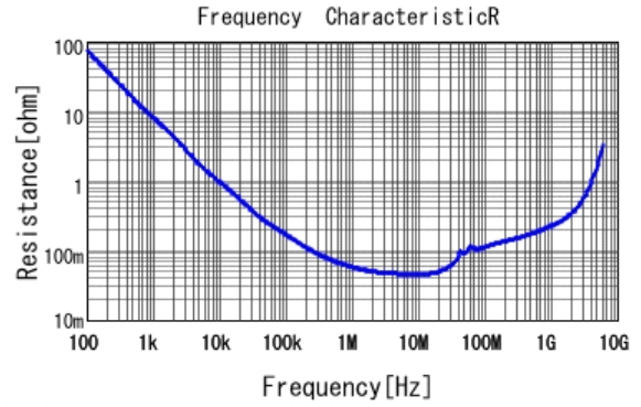
■ GCJ188R71H104MA12 R DCOV, 25degC
