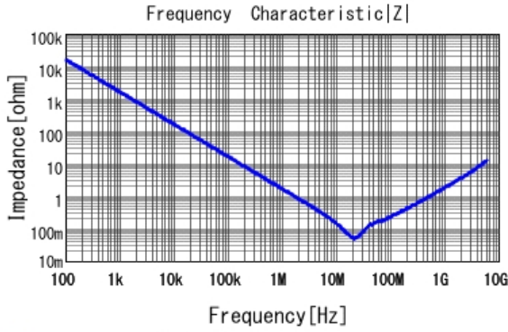
■ GCJ188R71H104MA12 |Z| DCOV, 25degC
