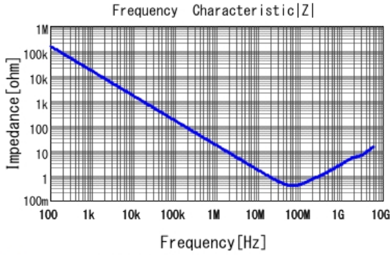
■ GCJ188R71C103KA01 |Z| DCOV, 25degC
