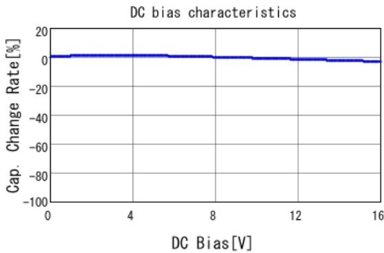
■ GCJ188R71C103KA01 C-DC bias capchange, 25.0degC, AC1.
