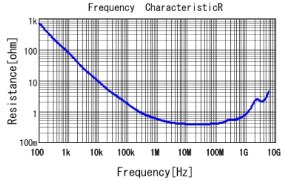
■ GCJ188R71C103KA01 R DCOV, 25degC
