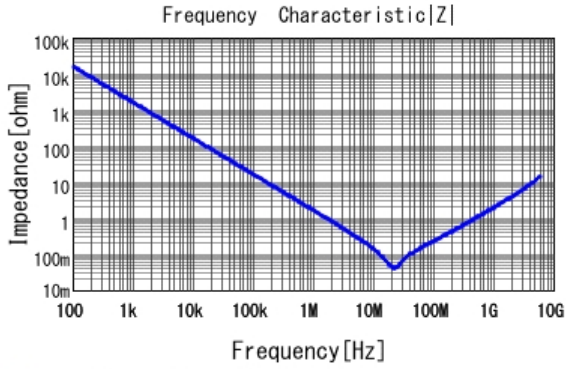
■ GCJ188L8EL104KA07 |Z| DC0V, 25degC
