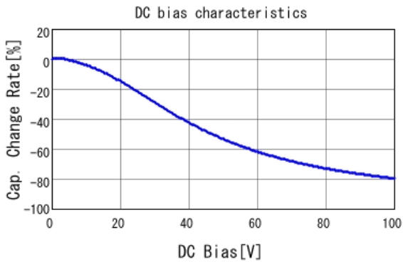
■ GCJ188L8EL104KA07 C-DC bias capchange, 25.0degC, AC1.
