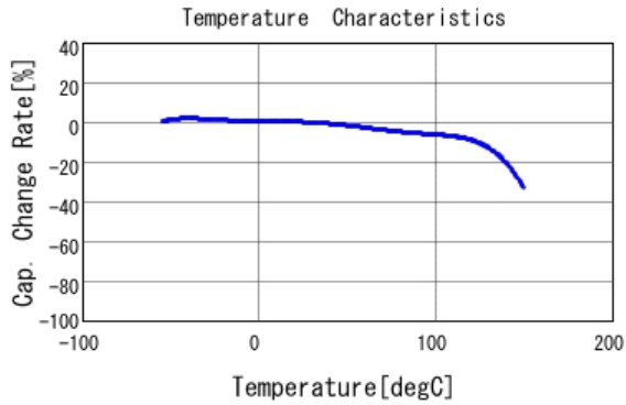
■ GCJ188L8EL104KA07 C-Temp. capchange, DC0.0V, AC1.0Vrm
