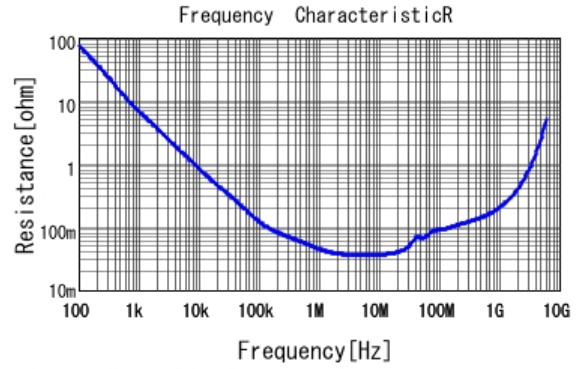
■ GCJ188L8EL104KA07 R DC0V, 25degC
