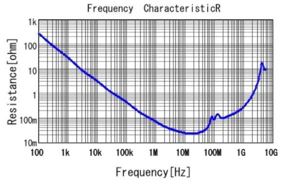
■ GCD21BR71H333MA01 R DCOV, 25degC
