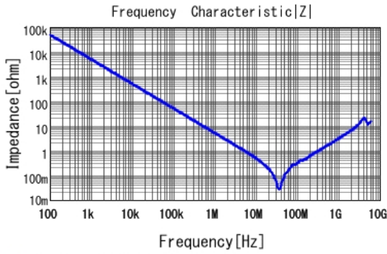
■ GCD21BR71H333MA01 |Z| DCOV, 25degC
