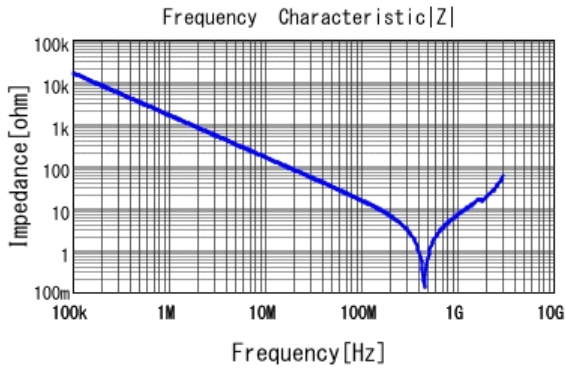
■ GA352QR7GF101KW31 |Z| DCOV, 25degC
