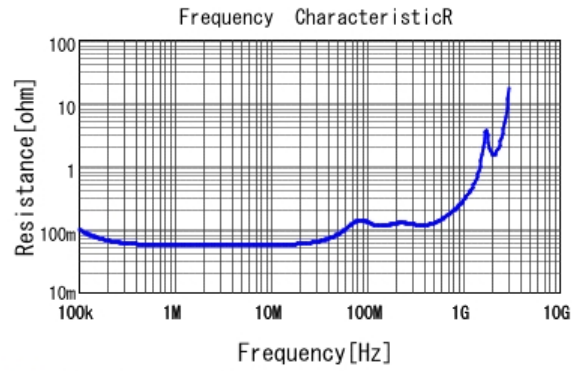
■ GA352QR7GF101KW31 R DCOV, 25degC
