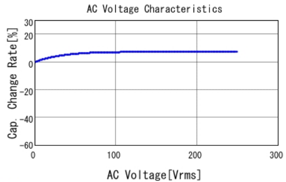
■ GA342QR7GD101KW01 C-AC Voltage capchange, DCOV, 25.0d
