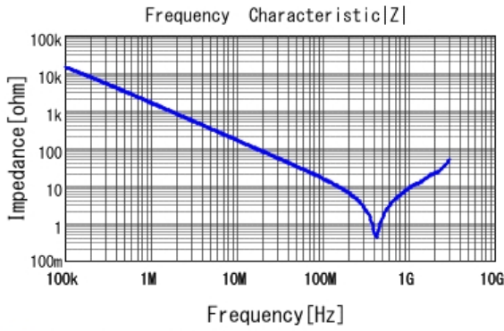
■ GA342QR7GD101KW01 |Z| DCOV, 25degC
