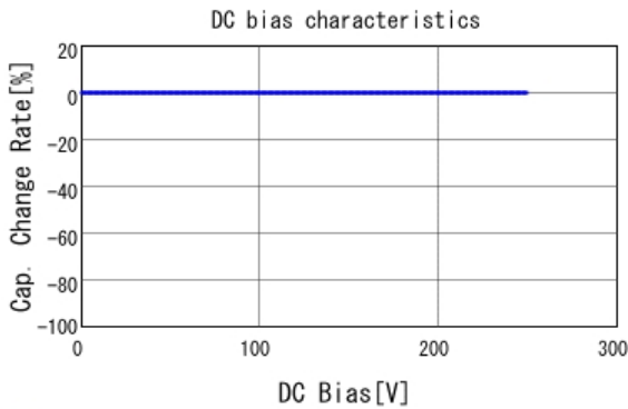
■ GA342QR7GD101KW01 C-DC bias capchange, 25.0degC, AC1V
