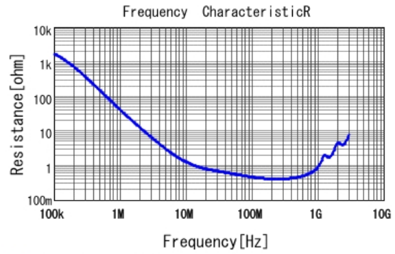
■ GA342QR7GD101KW01 R DCOV, 25degC
