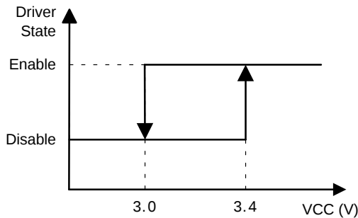
Figure 27. UVLO
