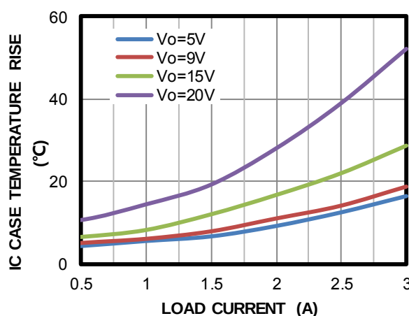
Thermal Rise
