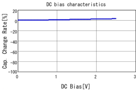
■ ECASD60E477M4R5K00 C-DC bias capchange, 25.0degC, AC1
