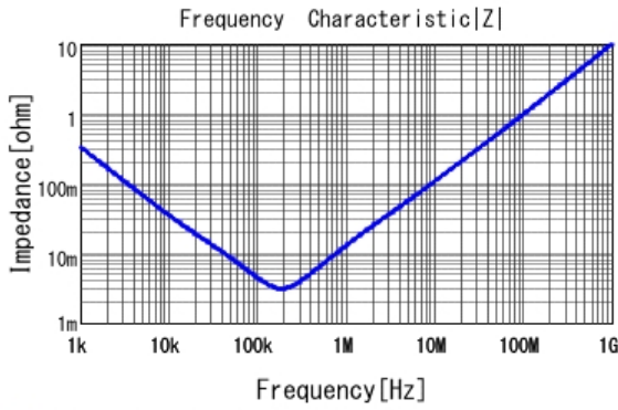
■ ECASD60E477M4R5K00 |Z| DCOV, 25degC
