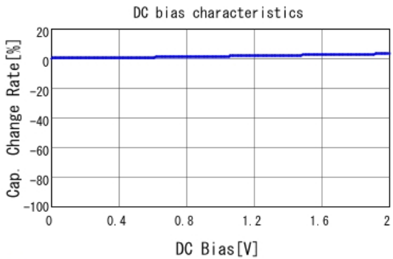
■ ECASD60D477M4R5K00 C-DC bias capchange, 25.0degC, AC1
