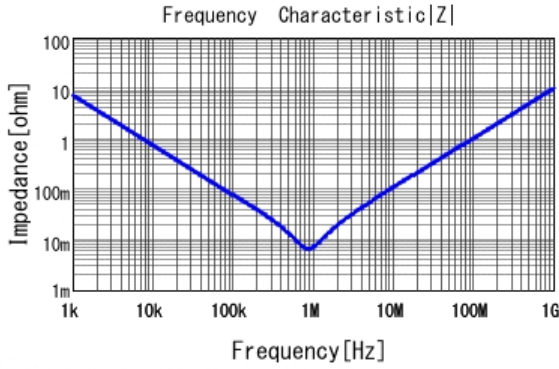
■ ECASD41E226M040KA0 |Z| DCOV, 25degC
