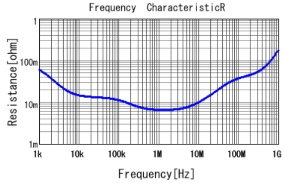
■ ECASD41E226M040KA0 R DCOV, 25degC
