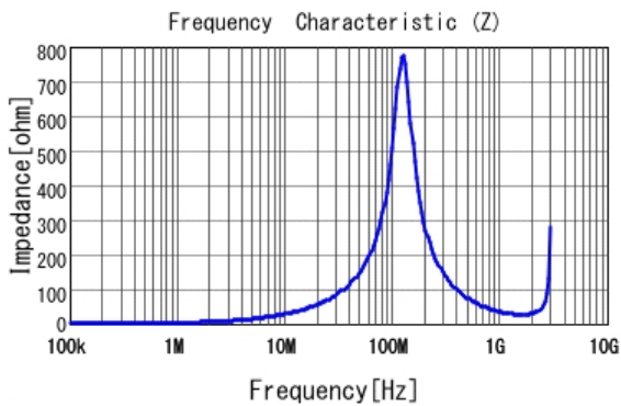
DFE2HCAHR47MJ0 |Z|
