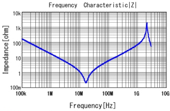
■ DE2F3KY103MA3BU02F |Z| DCOV, 20degC
