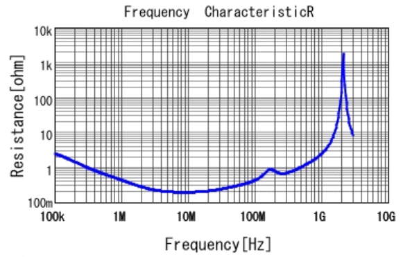
■ DE2F3KY103MA3BU02F R DCOV, 20degC
